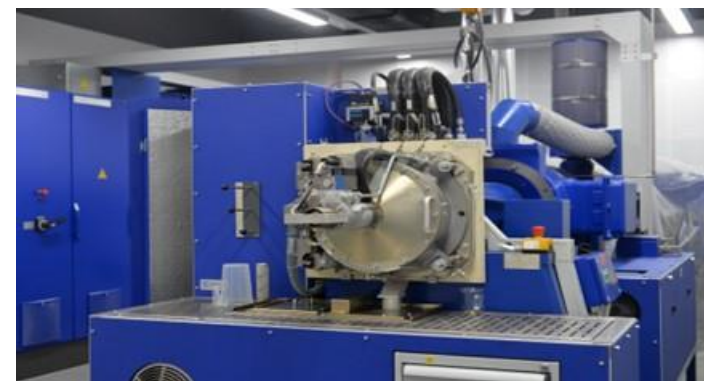
台架设备 GK Test Machine
